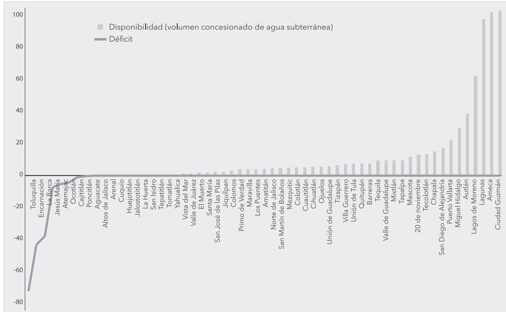
Gráfico 4.2. Disponibilidad del agua subterránea
