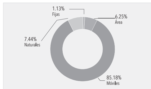
Gráfico 2.2. Porcentaje de emisiones a la atmósfera por tipo de fuente
