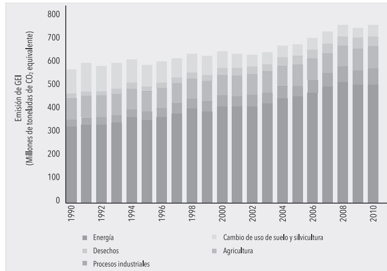
Gráfico 3.2. Emisión de GEI en México 1990-2010
